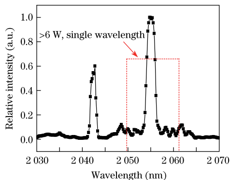
Fig. 5. Output spectrum of the composite Tm, Ho:YVO 4 laser.
