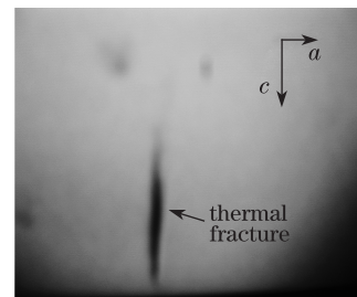
Fig. 4. Thermal fracture of the non-composite Tm, Ho:YVO 4 crystal.
